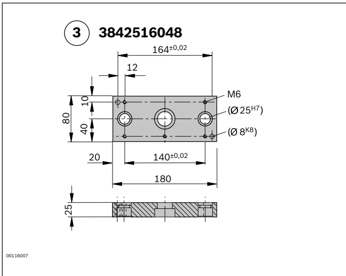
3 Hubplatte
