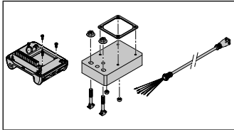
Anschlusseinheit Anbausatz Anschlusskabel
