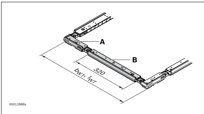
A Eckmodul B Verlängerungsmodul
