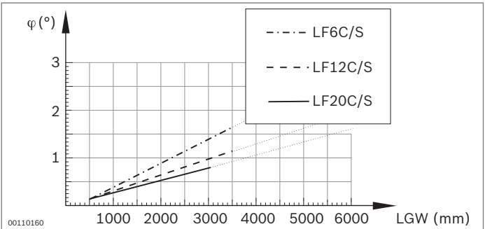
Diagramm 5: Verdrehwinkel
