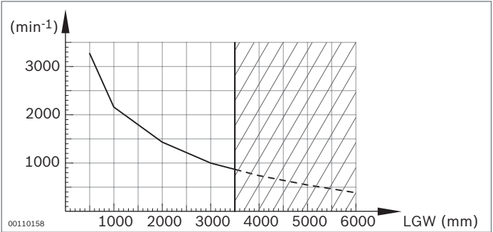
Diagramm 4: Lateralversatz
